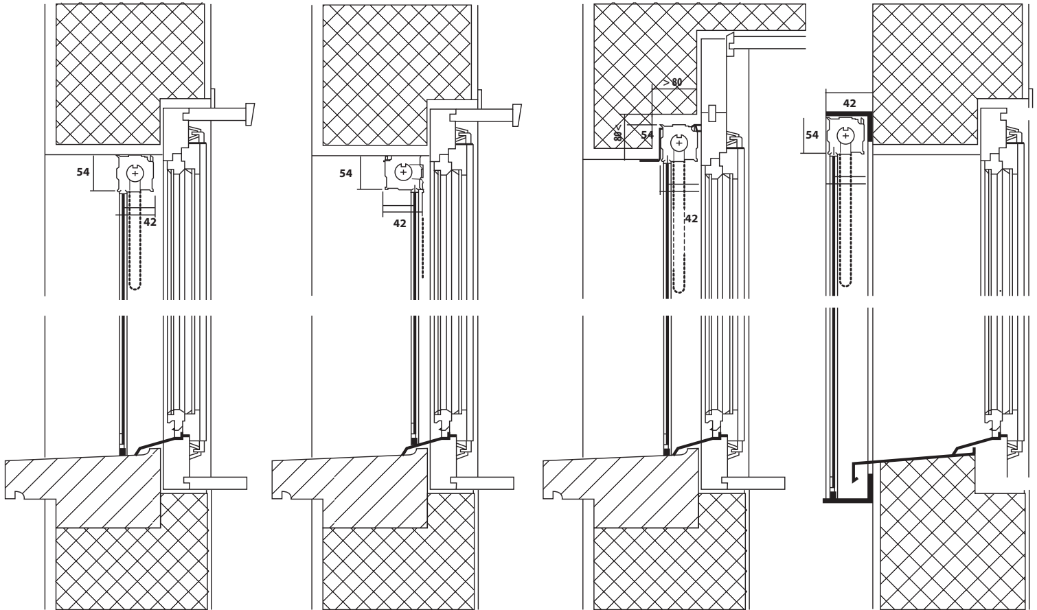
Abbildung 1 Einbau unter Abdeckung, normale Aufrollung, Kette links oder rechts unter dem Gehäuse.
