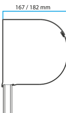
Caisson MONOBLOC type arrondi
