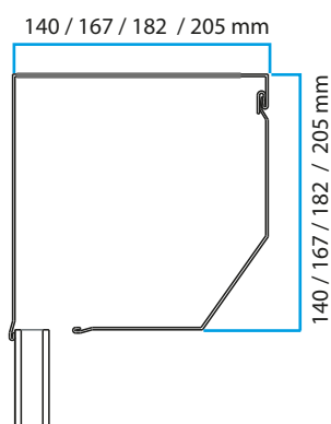
Caisson MONOBLOC type 45° (Standard)
