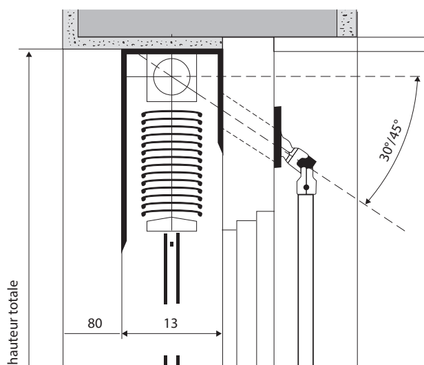
Coupe montage sous lambrequin
