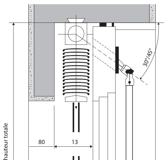
Coupe montage dans niche
